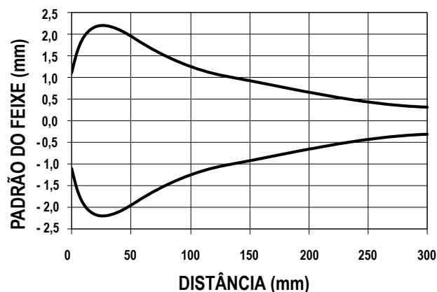
Figura 7: Padrão do Feixe
